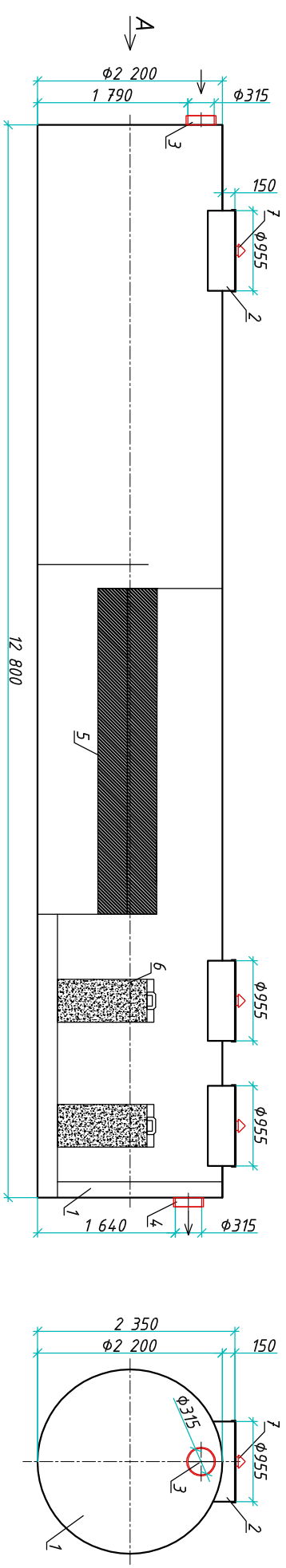
Разрез 1-1
